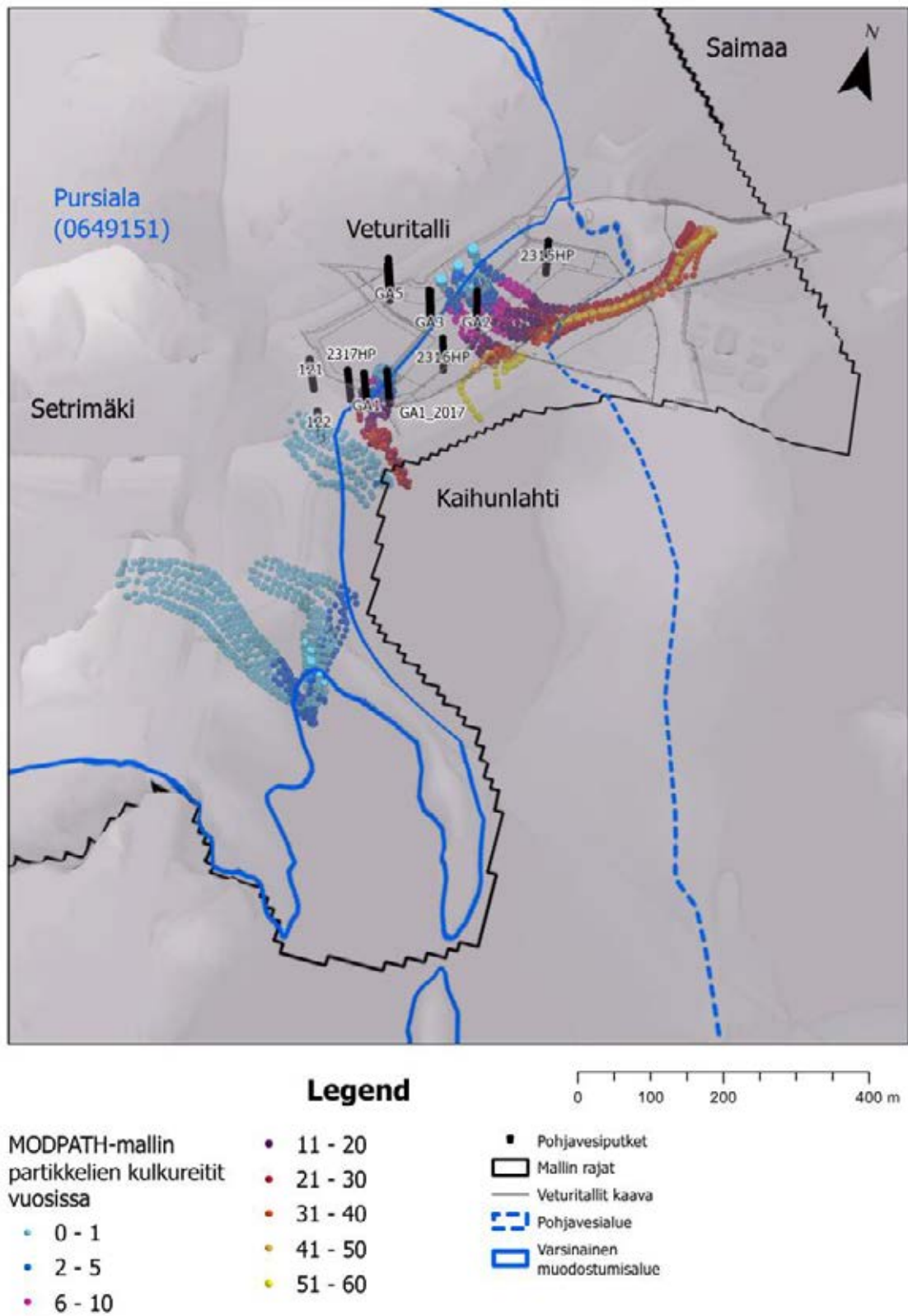
Kuva 4-3. MODPATH-mallin avulla mallinnettuja partikkelien kulkeutumisreitit ja kulkeutumisnopeudet kalibroidusta pohjavesimallista. Partikkelin kulkeutumisreitti kuvastaa pohjaveden kulkureittejä, joista advektion mukana kulkeutuvat haitta-aineet voivat kulkeutua.
