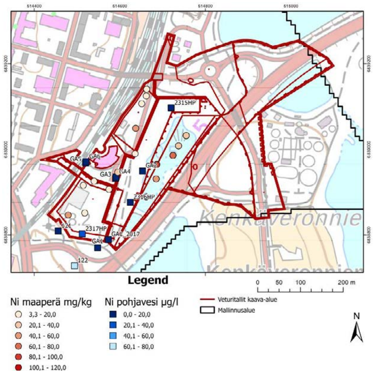
Kuva 3-7. Veturitallialueen nikkelihavainnot pohjavedessä ja maaperässä. Pohjaveden pitoisuudet ovat yksikössä µg/l ja maaperän mg/kg.
