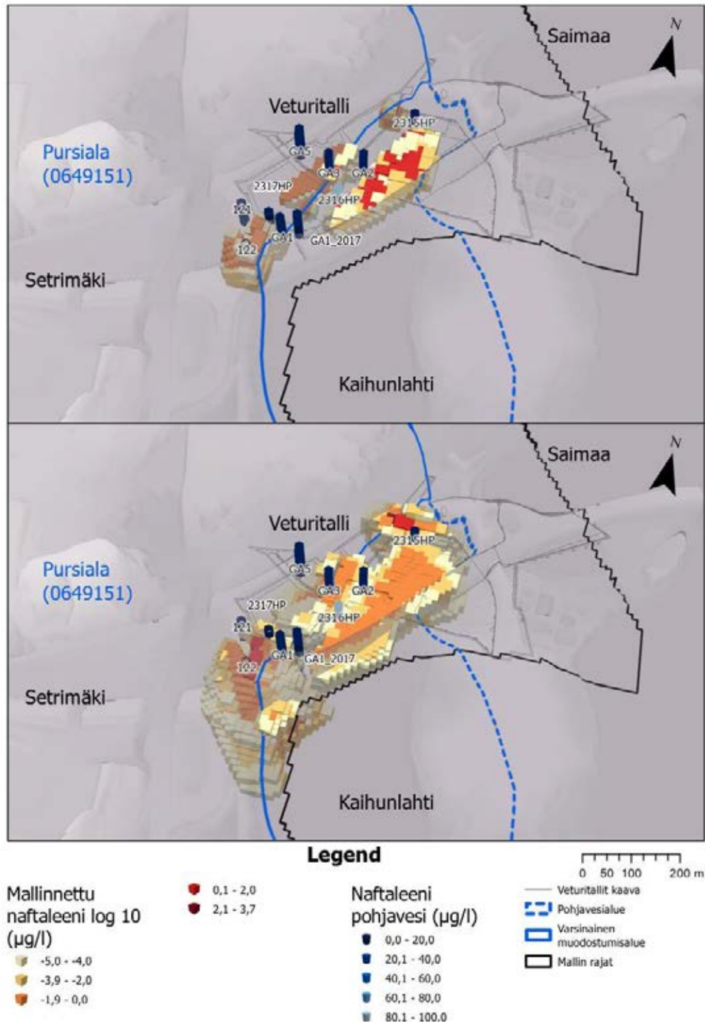
Kuva 4-20. Naftaleenin pitoisuudet lopputilanteen kuljetusmallin lähtötilassa (yllä). Naftaleenin mallinnettu kulkeutuminen 60 vuoden kuluttua lopputilanteesta massanvaihdon tilanteen mallissa (alla). Kuvan yksiköt ovat µg/l. Mallinnetut pitoisuudet ovat esitetty log10-muodossa niin, että esim. 3,0 vastaa arvoa 1000 µg/l ja maksimiarvo on 4940 µg/l. Vastaavasti -5 tarkoittaa pitoisuutta 0,00001 µg/l.
