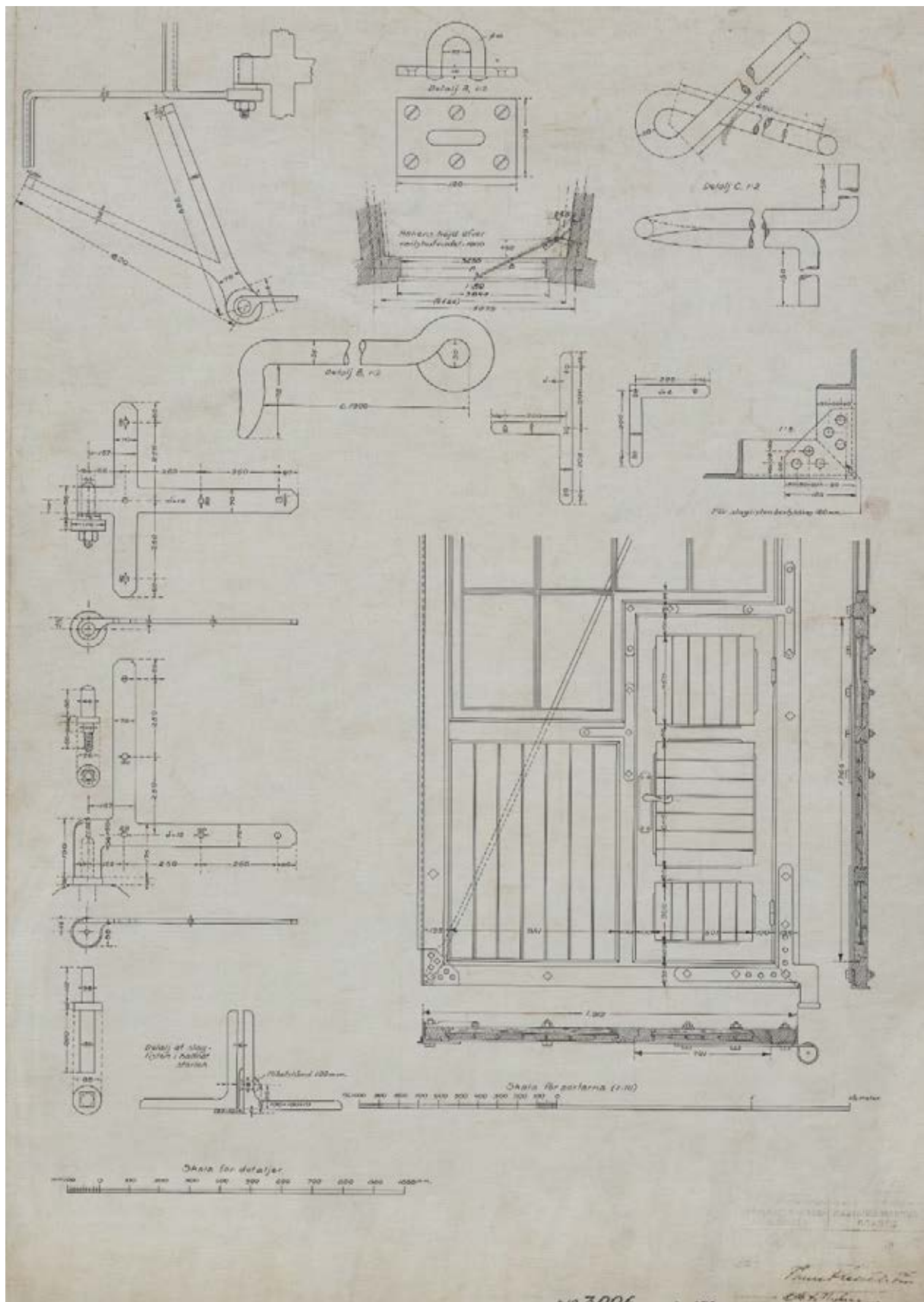
Kuva 49. Detaljipiirustus tallinovista 1 ja 2 ilmeisesti vuodelta 1915. Lähde: Kansallisarkisto.
