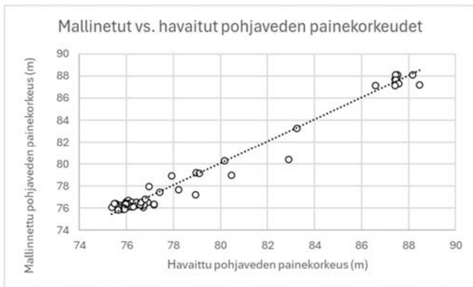
Kuva 4-2. Pistekaavio mallinnettujen ja havaittujen pohjaveden painekorkeuksien eroista kalibroidussa mallissa.
