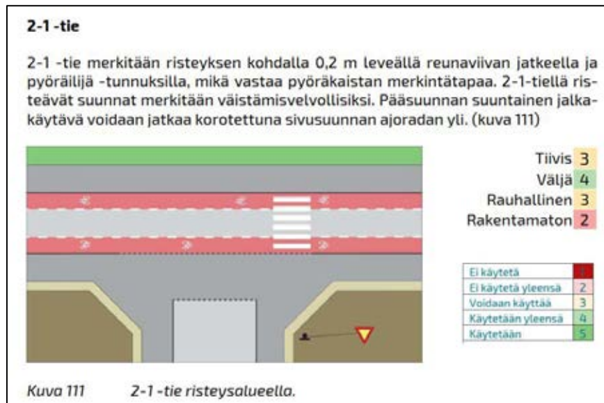
Kuva 18. Ote Pyöräliikenteen suunnitteluohjeesta 2-1 -tiestä. Lähde: Pyöräliikenteen suunnitteluohje, Väyläviraston ohjeita 18/2020.
