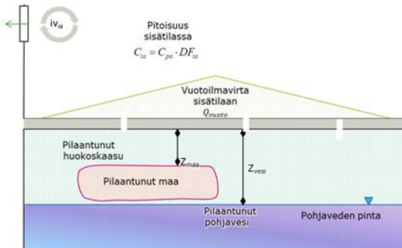
Kuva 1. Yksinkertaistettu malli haitta-aineiden kulkeutumisesta huokosilmasta rakennuksen alustatilaan
