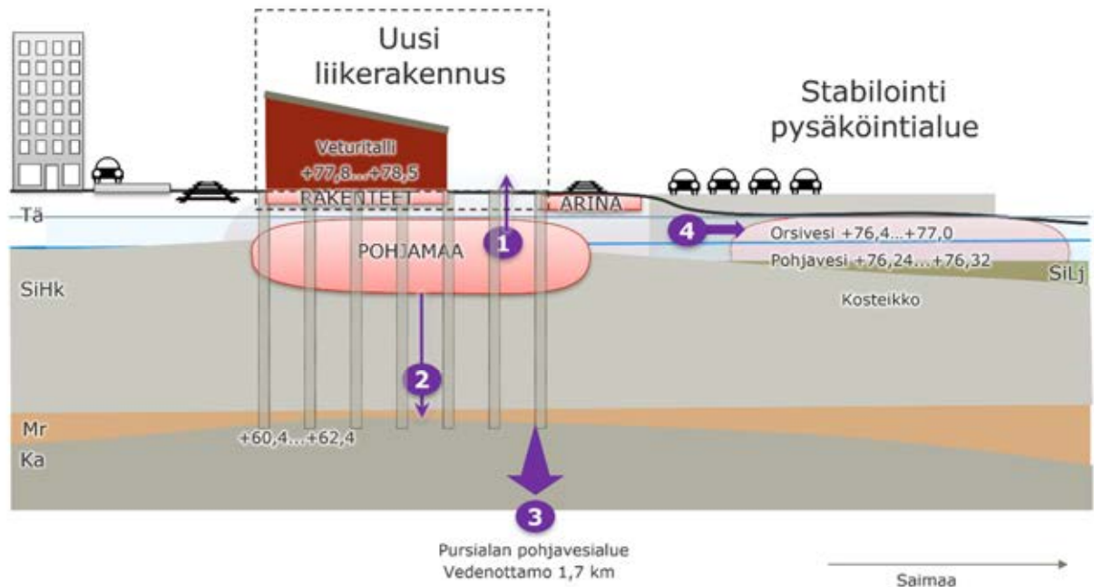
Kuva 2 Käsitteellinen malli. Pysäköintialue rakennetaan joko stabiloimalla tai louhepenkereellä.
