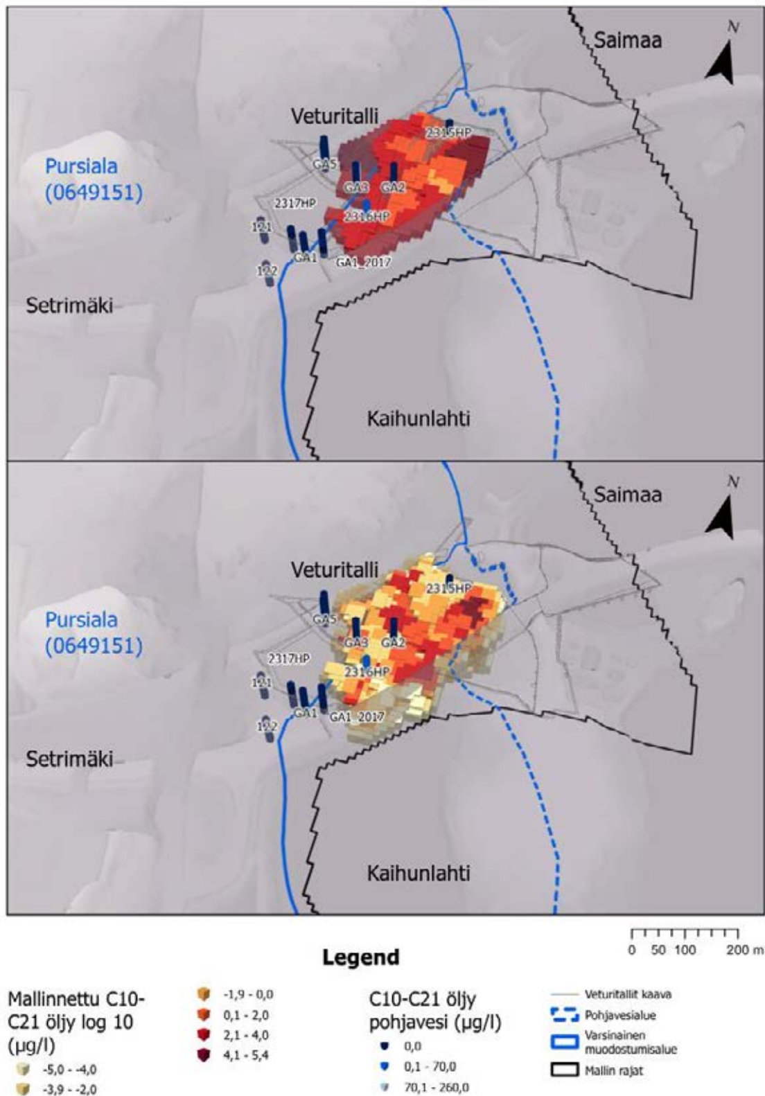
Kuva 4-11. Öljyn jakeen C10-C21 pitoisuudet kuljetusmallin lähtötilassa (yllä). C10-C21 öljyn jakeen mallinnettu kulkeutuminen 60 vuoden kuluttua lähtötilanteesta (alla). Kuvan yksiköt ovat µg/l. Mallinnetut pitoisuudet ovat esitetty log10-muodossa niin, että esim. 4,0 vastaa arvoa 10000 µg/l ja maksimiarvo on 280000 µg/l eli 280 mg/l. Vastaavasti -5 tarkoittaa pitoisuutta 0,00001 µg/l.
