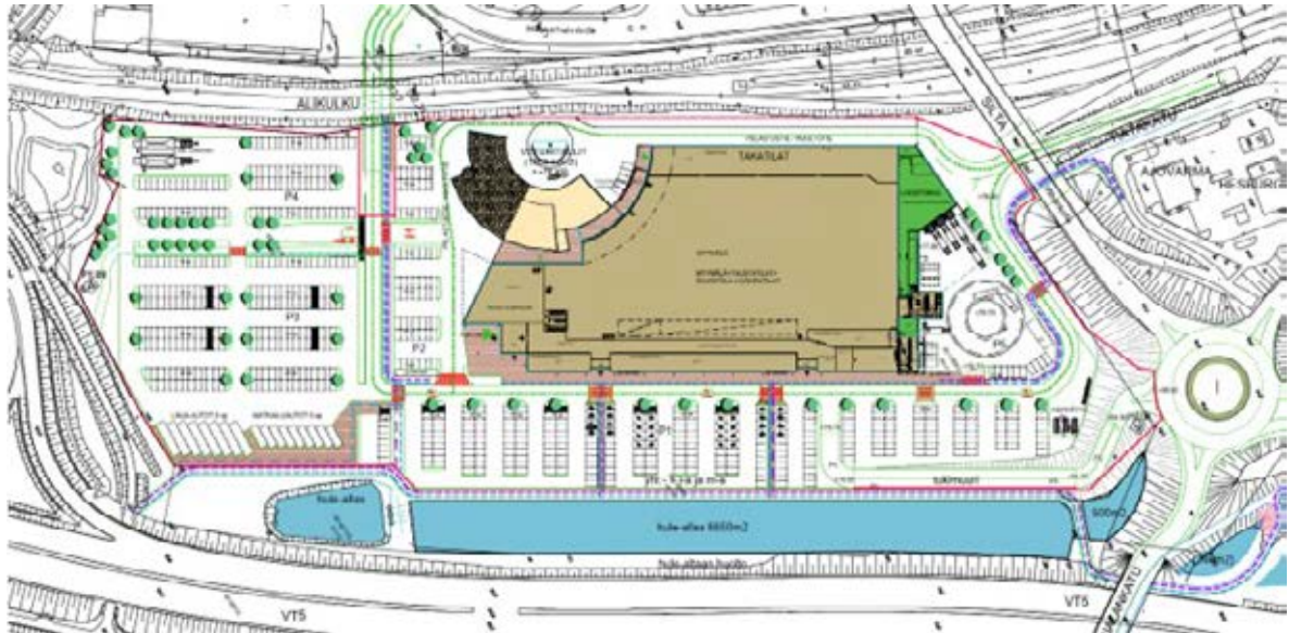
Kuva 29. Ote Arkkitehtitoimisto Ark'idea Oy:n tontinkäyttösuunnitelmasta.
