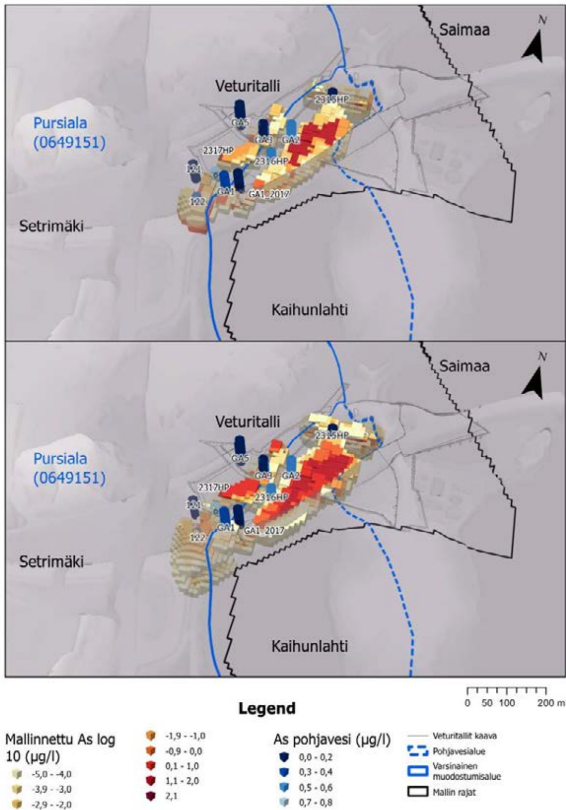
Kuva 4-13. Arseenin pitoisuudet massanvaihdon kuljetusmallin lähtötilassa (yllä). Arseenin kulkeutuminen sorption kanssa mallinnettuna 60 vuoden kuluttua lähtötilanteesta massanvaihdon tilanteen mallissa (alla). Kuvan yksiköt ovat \mu\text{g/l} . Mallinnetut pitoisuudet ovat esitetty log 10 -muodossa niin, että esim. 2,0 vastaa arvoa 100 \mu\text{g/l} ja maksimiarvo on 122 \mu\text{g/l} . Vastaavasti -5 tarkoittaa pitoisuutta 0,00001 \mu\text{g/l} .
