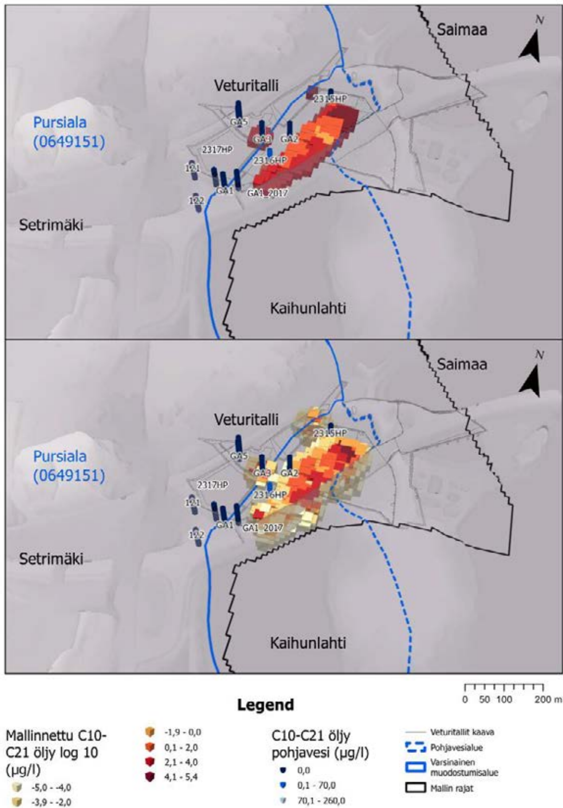
Kuva 4-18. C10-C21 öljyjakeiden pitoisuudet massanvaihdon kuljetusmallin lähtötilassa (yllä). C10-21 öljyjakeiden mallinnettu kulkeutuminen 60 vuoden kuluttua massanvaihdon tilanteen mallissa (alla). Kuvan yksiköt ovat µg/l. Mallinnetut pitoisuudet ovat esitetty log10-muodossa niin, että esim. 4,0 vastaa arvoa 10000 µg/l ja maksimiarvo on 280000 µg/l eli 280 mg/l. Vastaavasti -5 tarkoittaa pitoisuutta 0,00001 µg/l.
