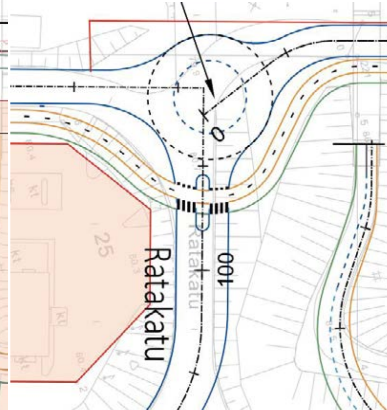
Kuva 17. Yliajettava liikenneympyrä.
