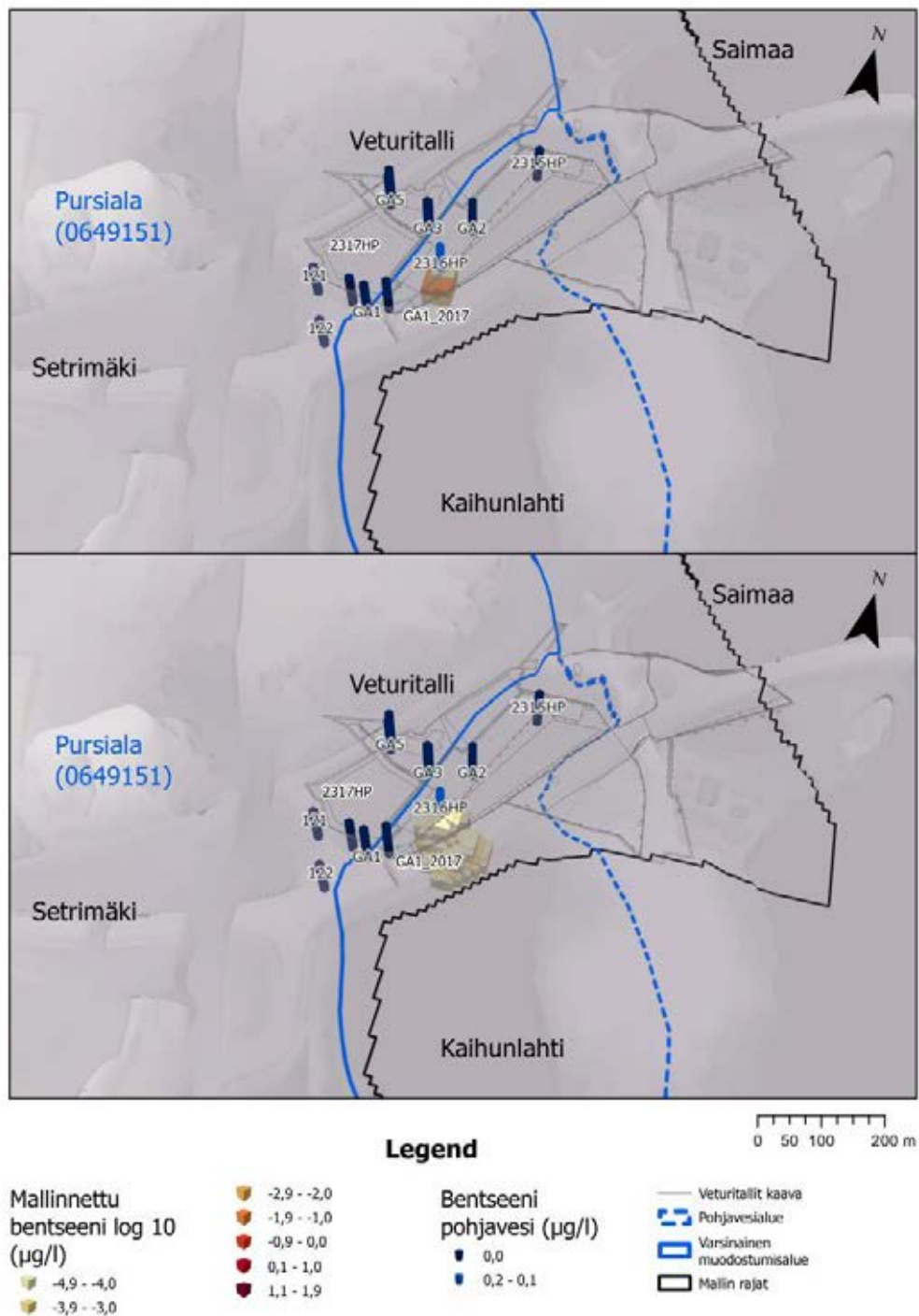
Kuva 4-15. Bentseenin pitoisuudet massanvaihdon kuljetusmallin lähtötilassa (yllä). Bentseenin mallinnettu kulkeutuminen 60 vuoden kuluttua lähtötilanteesta massanvaihdon tilanteen mallissa (alla). Kuvan yksiköt ovat \mu\text{g/l} . Mallinnetut pitoisuudet ovat esitetty log10-muodossa niin, että esim. 1,0 vastaa arvoa 10 \mu\text{g/l} ja maksimiarvo on 80,9 \mu\text{g/l} . Vastaavasti -5 tarkoittaa pitoisuutta 0,00001 \mu\text{g/l} .
