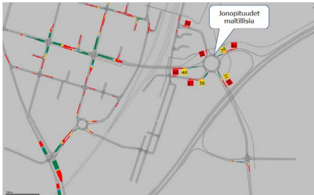
Kuva 38. Jonopituudet IHT, kiertoliittymä 5-haaraa. (Ramboll, 2026).
