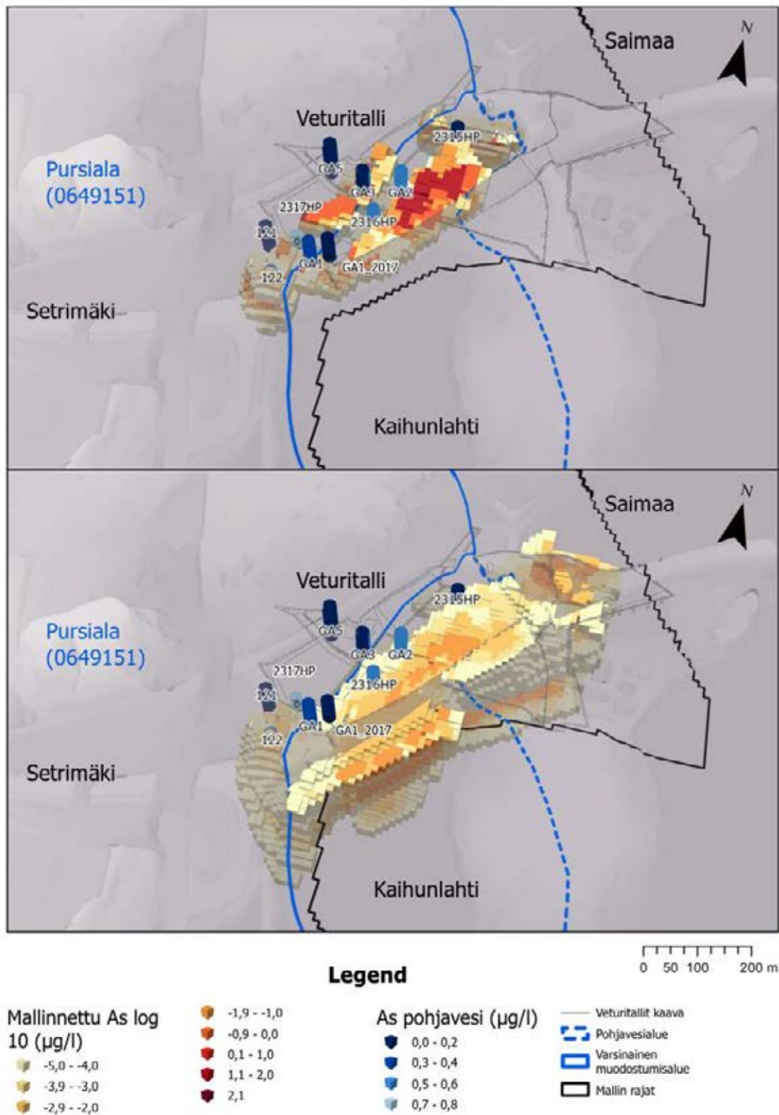
Kuva 4-14. Arseenin pitoisuudet massanvaihdon kuljetusmallin lähtötilassa ilman sorptiota (yllä). Arseenin kulkeutuminen ilman sorptiota mallinnettuna 60 vuoden kuluttua lähtötilanteesta massanvaihdon tilanteen mallissa (alla). Kuvan yksiköt ovat µg/l. Mallinnetut pitoisuudet ovat esitetty log10-muodossa niin, että esim. 2,0 vastaa arvoa 100 ja maksimiarvo on 122 µg/l. Vastaavasti -5 tarkoittaa pitoisuutta 0,00001 µg/l.
