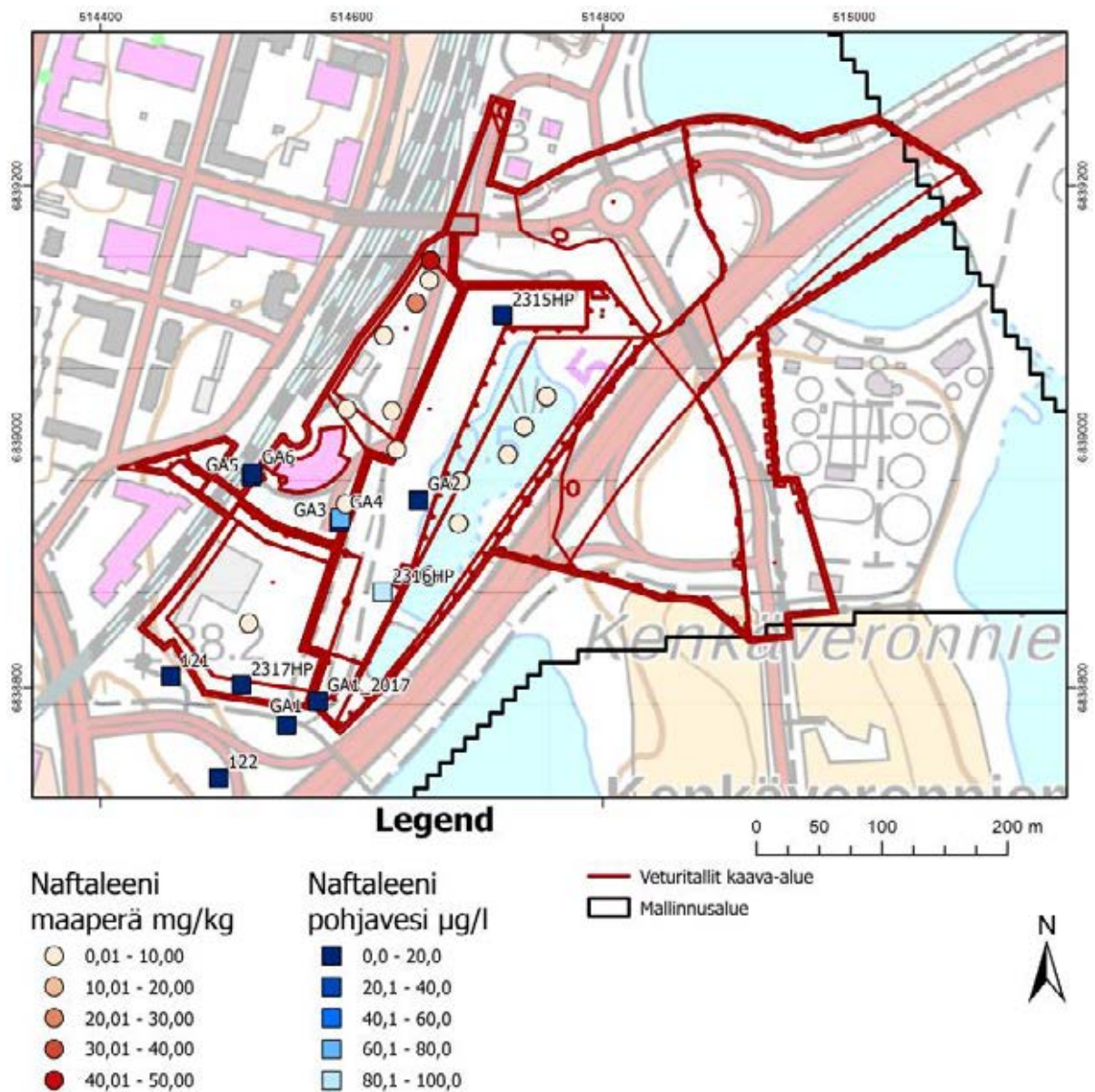
Kuva 3-6. Naftaleeni esiintyminen pohjavedessä ja maaperässä. Pohjaveden pitoisuudet ovat yksikössä µg/l ja maaperän mg/kg.
