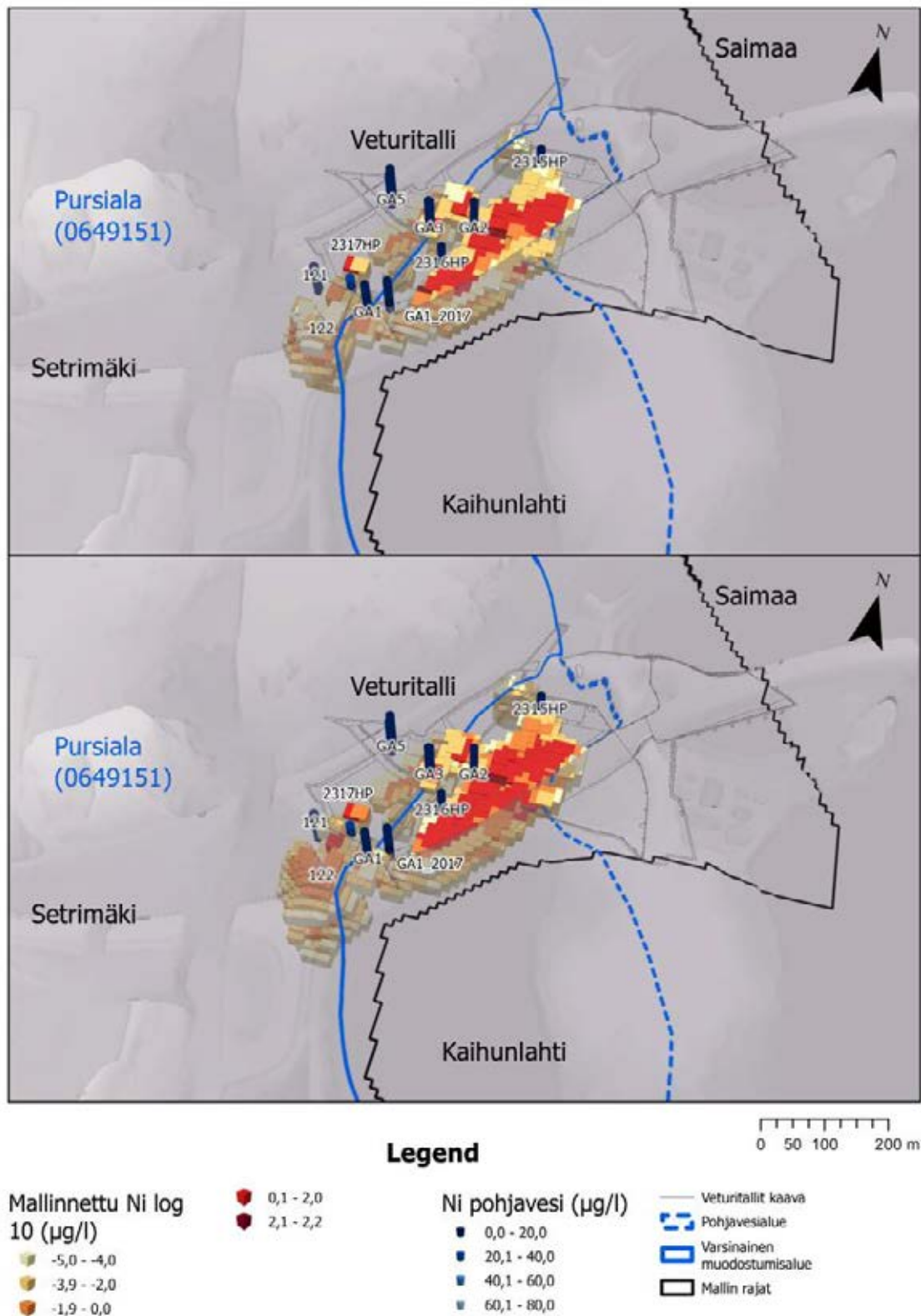
Kuva 4-17. Nikkelin pitoisuudet massanvaihdon kuljetusmallin lähtötilassa (yllä). Nikkelin mallinnettu kulkeutuminen 60 vuoden kuluttua massanvaihdon tilanteen mallissa (alla). Kuvan yksiköt ovat µg/l. Mallinnetut pitoisuudet ovat esitetty log10-muodossa niin, että esim. 2,0 vastaa arvoa 100 µg/l ja maksimi-arvo on 170 µg/l. Vastaavasti -5 tarkoittaa pitoisuutta 0,00001 µg/l.
