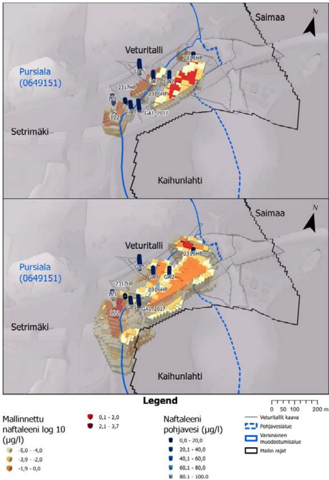
Kuva 4-16. Naftaleenin pitoisuudet massanvaihdon kuljetusmallin lähtötilassa (yllä). Naftaleenin mallinnettu kulkeutuminen 60 vuoden kuluttua massanvaihdon tilanteen mallissa (alla). Kuvan yksiköt ovat µg/l. Mallinnetut pitoisuudet ovat esitetty log10-muodossa niin, että esim. 3,0 vastaa arvoa 1000 µg/l ja maksimi-arvo on 4940 µg/l. Vastaavasti -5 tarkoittaa pitoisuutta 0,00001 µg/l.
