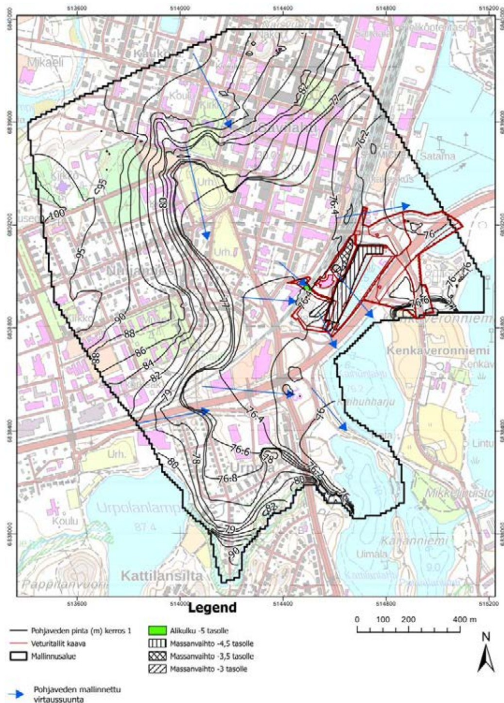
Kuva 4-5. Pohjaveden virtaussuunnat lopputilanteen mallissa kerros 1:sta kuvattuna pohjaveden korkeuskäyrinä ja virtausnuolina (siniset nuolet).
