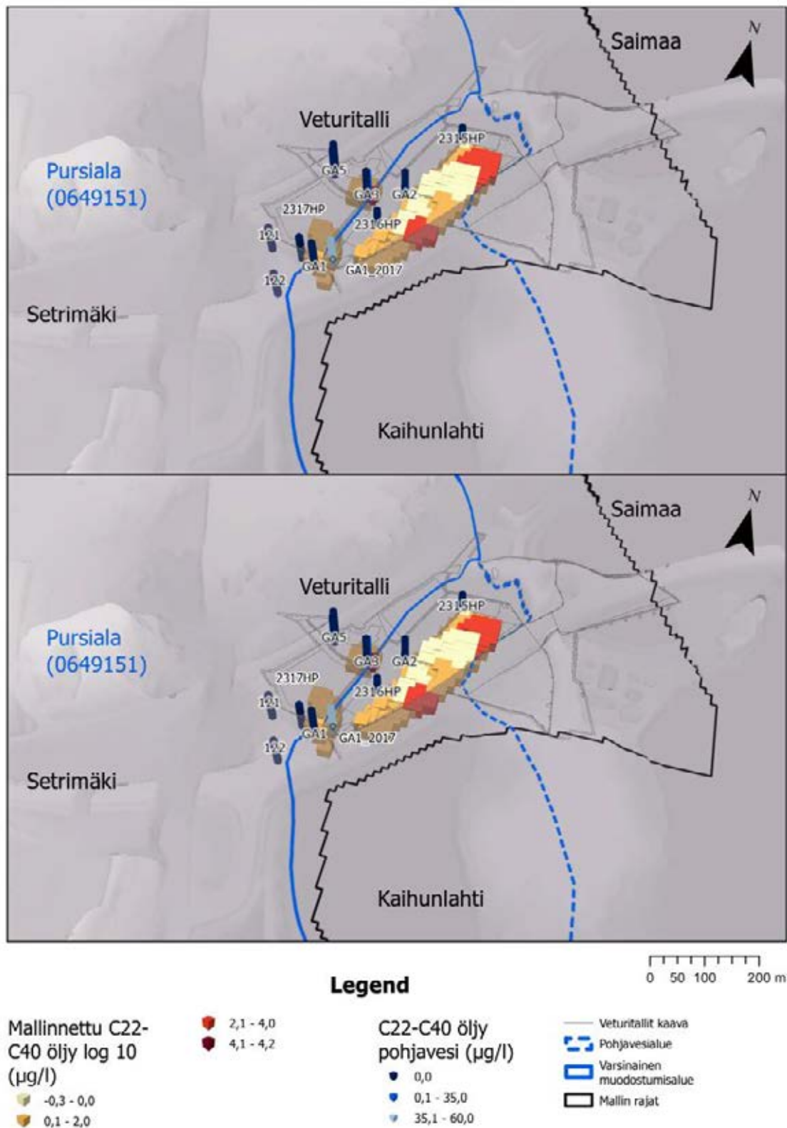
Kuva 4-19. C22-C40 öljyjakeiden pitoisuudet massanvaihdon kuljetusmallin lähtötilassa (yllä). C22-40 öljyjakeiden mallinnettu kulkeutuminen 60 vuoden kuluttua massanvaihdon tilanteen mallissa (alla). Kuvan yksiköt ovat µg/l. Mallinnetut pitoisuudet ovat esitetty log10-muodossa niin, että esim. 4,0 vastaa arvoa 10000 µg/l ja maksimiarvo on 15200 µg/l eli 152 mg/l. Vastaavasti -5 tarkoittaa pitoisuutta 0,00001 µg/l.
