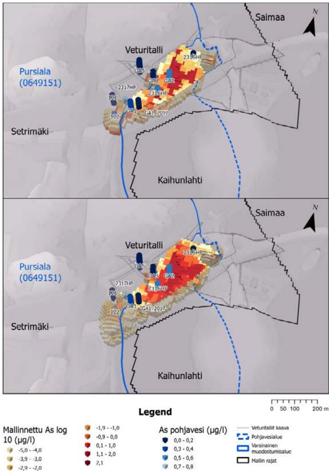
Kuva 4-6. Arseenin pitoisuudet kuljetusmallin lähtötilassa (yllä). Arseenin mallinnettu kulkeutuminen sorption kanssa 60 vuoden kuluttua lähtötilanteesta (alla). Kuvan yksiköt ovat µg/l. Mallinnetut pitoisuudet ovat esitetty log10-muodossa niin, että esim. 2,0 vastaa arvoa 100 µg/l ja maksimiarvo on 122 µg/l. Vastaavasti -5 tarkoittaa pitoisuutta 0,00001 µg/l.
