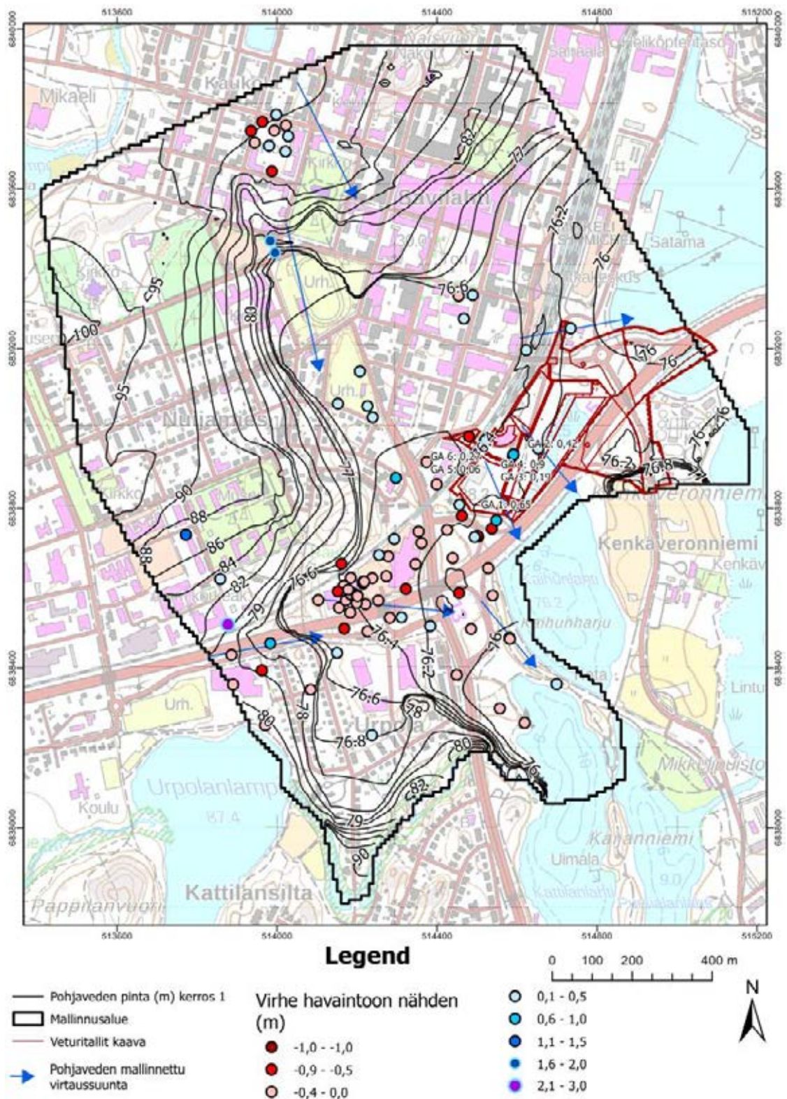
Kuva 4-1. Mallinnetut pohjaveden virtaussuunnat alkutilan mallissa esitettynä mallin laskentakerron 1:sta kuvattuna pohjaveden korkeuskäyrinä ja virtausnuolina (siniset nuolet). Pohjavesiputkien pisteissä positiiviset arvot (sinisävyt) kuvastavat, että mallinnettu pohjaveden painekorkeuden arvo on pienempi kuin havaittu arvo ja negatiiviset arvot (punäsävyt) kuvastavat alueita, jossa mallinnettu pohjaveden painekorkeus on korkeammalla kuin pohjavesiputkessa havaittu vesipinta.
