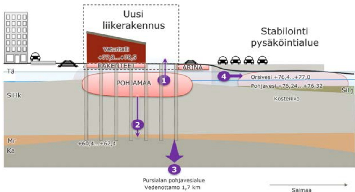
Kuva 1 Käsitteellinen malli. Pysäköintialue rakennetaan joko stabiloimalla tai louhepenkereellä.
