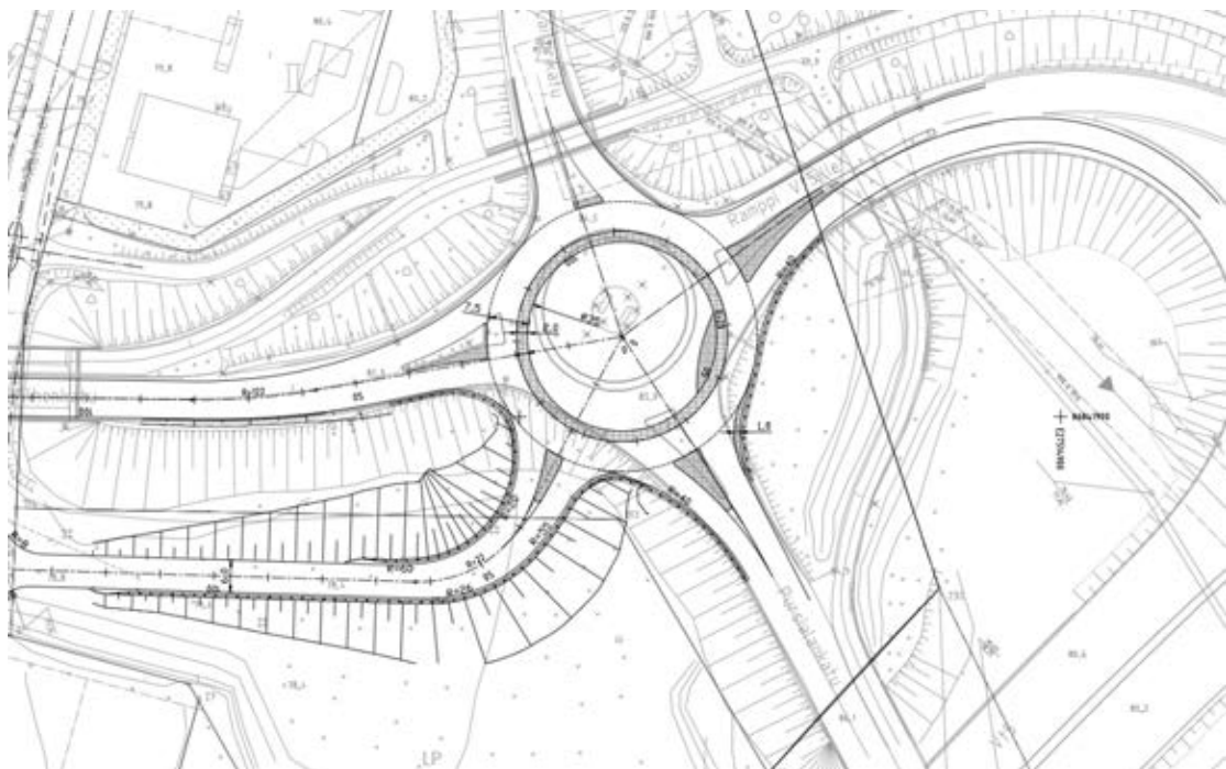
Kuva 41. Aseman kiertoliittymä ja viideshaara, Ramboll, 2025.
