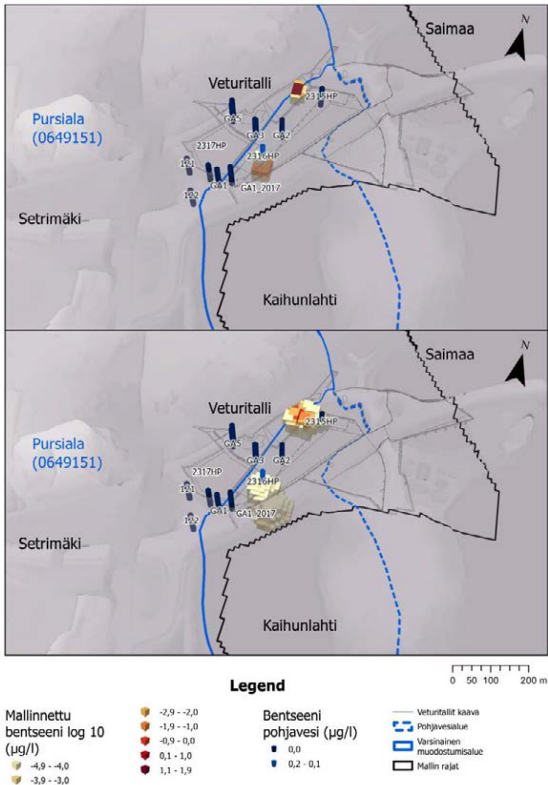
Kuva 4-8. Bentseenin pitoisuudet kuljetusmallin lähtötilassa (yllä). Bentseenin mallinnettu kulkeutuminen 60 vuoden kuluttua lähtötilanteesta (alla). Kuvan yksiköt ovat µg/l. Mallinnetut pitoisuudet ovat esitetty log10-muodossa niin, että esim. 1,0 vastaa arvoa 10 µg/l ja maksimiarvo on 80,9 µg/l. Vastaavasti -5 tarkoittaa pitoisuutta 0,00001 µg/l.
