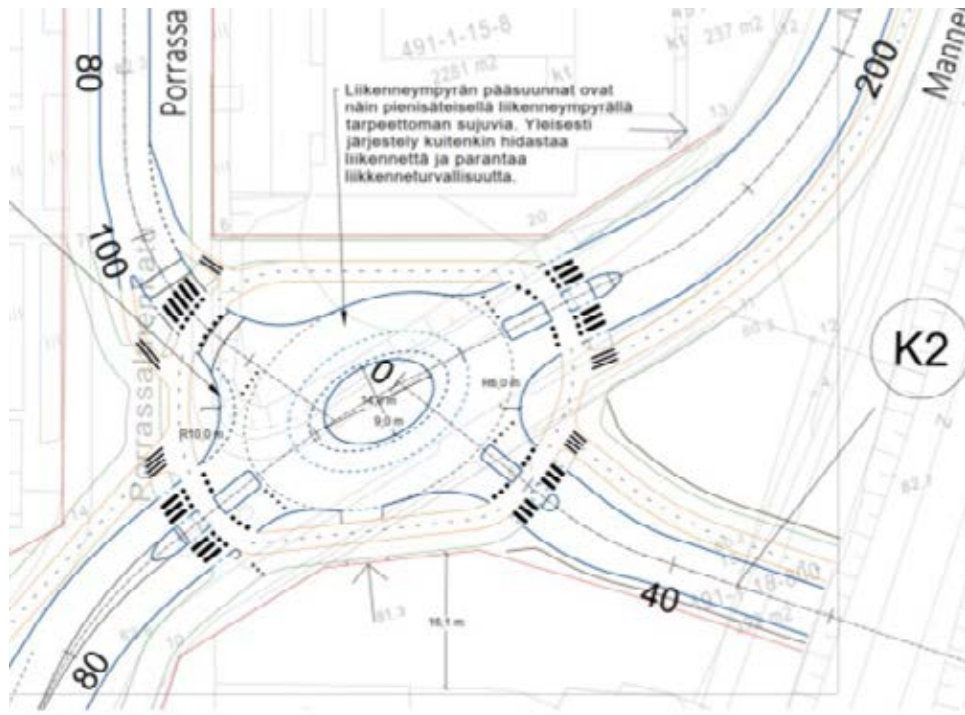
Kuva 40. Suunnitelmaluonnos Mannerheimintien soikion muotoisen liikenneympyrävaihtoehdon tilavaatimuksesta. (Sitowise Oyj, 2022)
