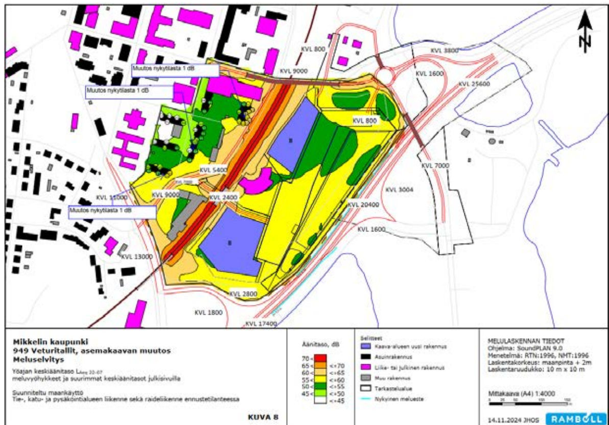
Kuva 42. Yöajan keskiäänitaso L_{Aeq} 22-07 , meluvyöhykkeet ja suurimmat keskiäänitasot julkisivuilla. Mallinnuksessa on huomioitu suunniteltu maankäyttö sekä tie-, katu- ja pysäköintialueen liikenne ja raideliikenne ennustetilanteessa (Ramboll, 2024).
