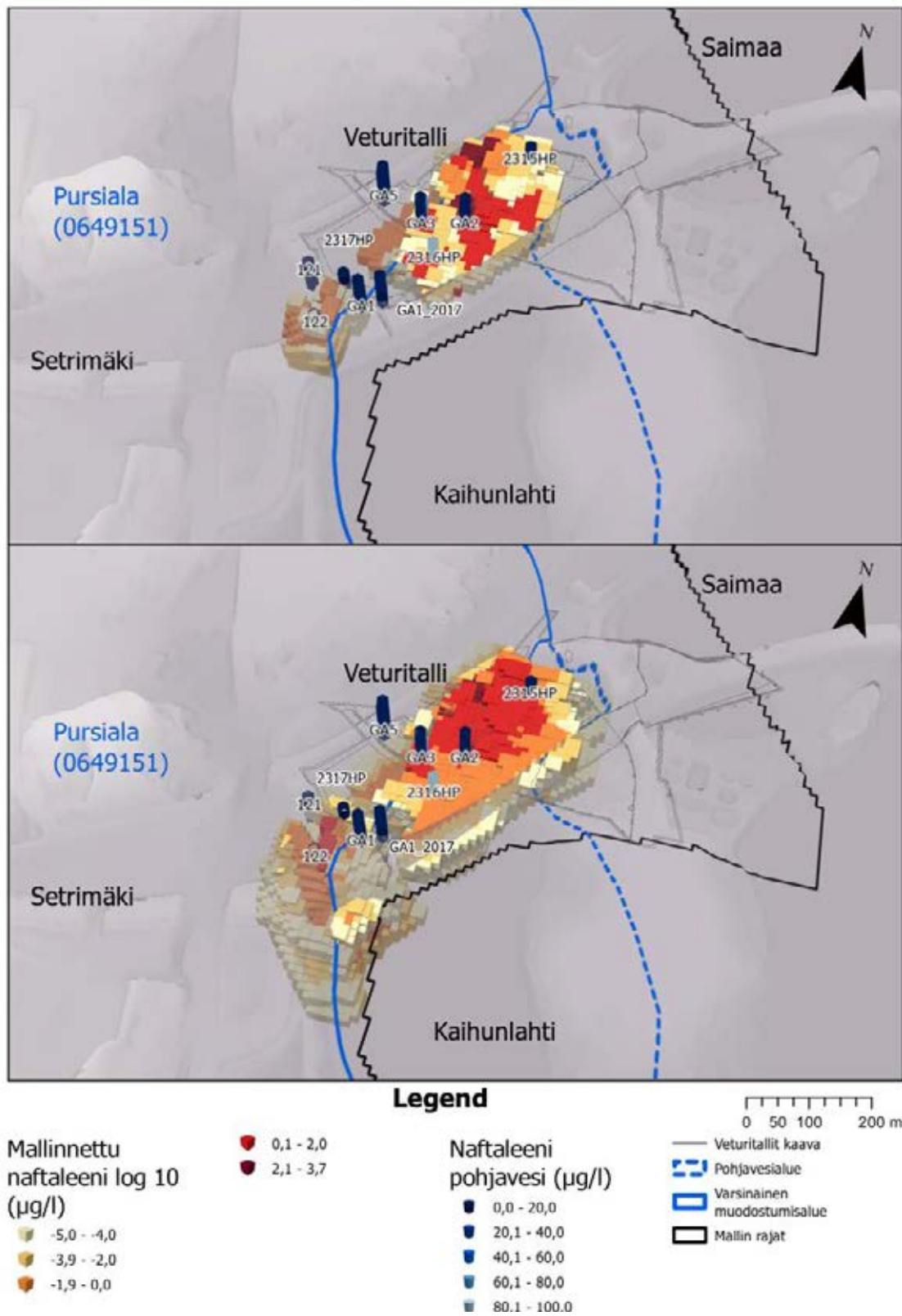
Kuva 4-9. Naftaleenin pitoisuudet kuljetusmallin lähtötilassa (yllä). Naftaleenin mallinnettu kulkeutuminen 60 vuoden kuluttua lähtötilanteesta (alla). Kuvan yksiköt ovat µg/l. Mallinnetut pitoisuudet ovat esitetty log10-muodossa niin, että esim. 3,0 vastaa arvoa 1000 µg/l ja maksimiarvo on 4940 µg/l. Vastaavasti -5 tarkoittaa pitoisuutta 0,00001 µg/l.
