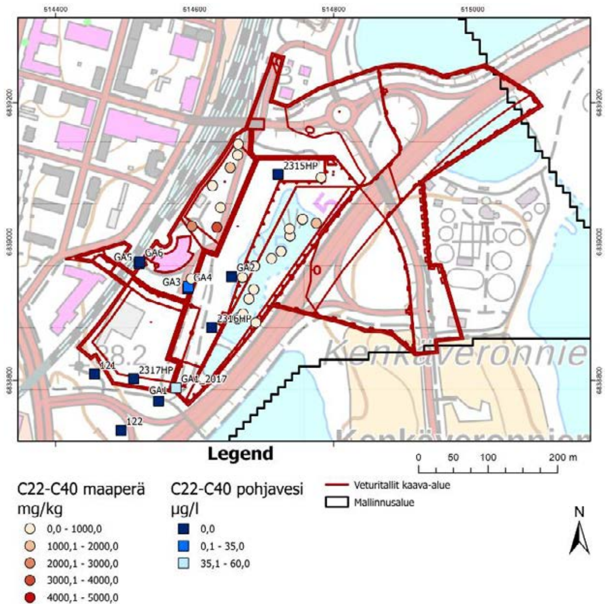
Kuva 3-9. Öljyn C22-C40 jakeen esiintyminen maaperässä ja pohjavedessä. Pohjaveden pitoisuudet ovat yksikössä µg/l ja maaperän mg/kg.
