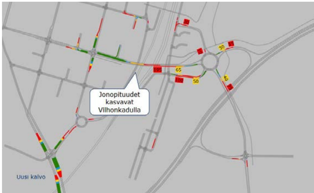
Kuva 39. Jonopituudet IHT, kiertoliittymä 5-haaraa, alikulkua ei vielä rakennettu. (Ramboll, 2026).
