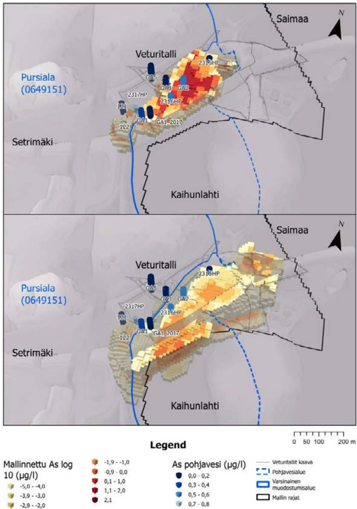
Kuva 4-7. Arseenin pitoisuudet kuljetusmallin lähtötilassa (yllä). Arseenin mallinnettu kulkeutuminen ilman sorptiota 60 vuoden kuluttua lähtötilanteesta (alla). Kuvan yksiköt ovat µg/l. Mallinnetut pitoisuudet ovat esitetty log10-muodossa niin, että esim. 2,0 vastaa arvoa 100 µg/l ja maksimiarvo on 122 µg/l. Vastaavasti -5 tarkoittaa pitoisuutta 0,00001 µg/l.
