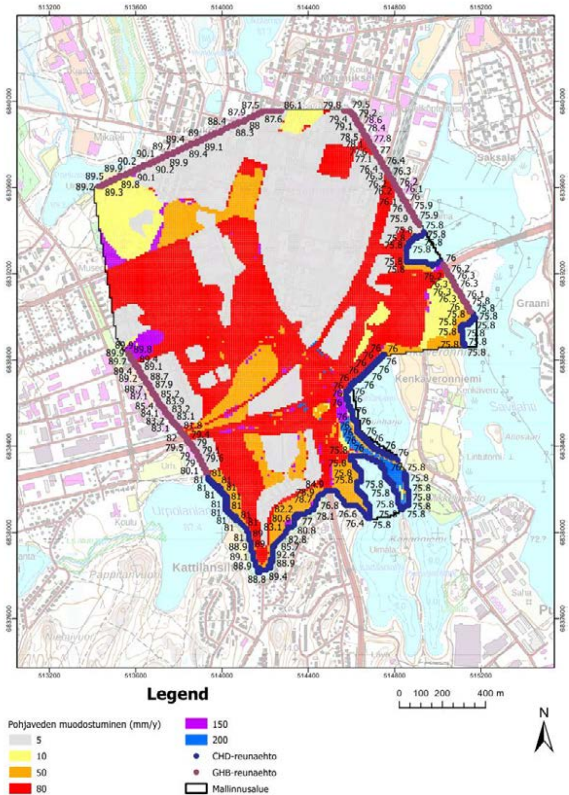
Kuva 3-2. Pohjavesimallin reunaehdot. CHD- ja GHB-reunaehto- jen määritetyt pohjavedenpinnan painetasot ovat esitetty kuvassa metreinä.
