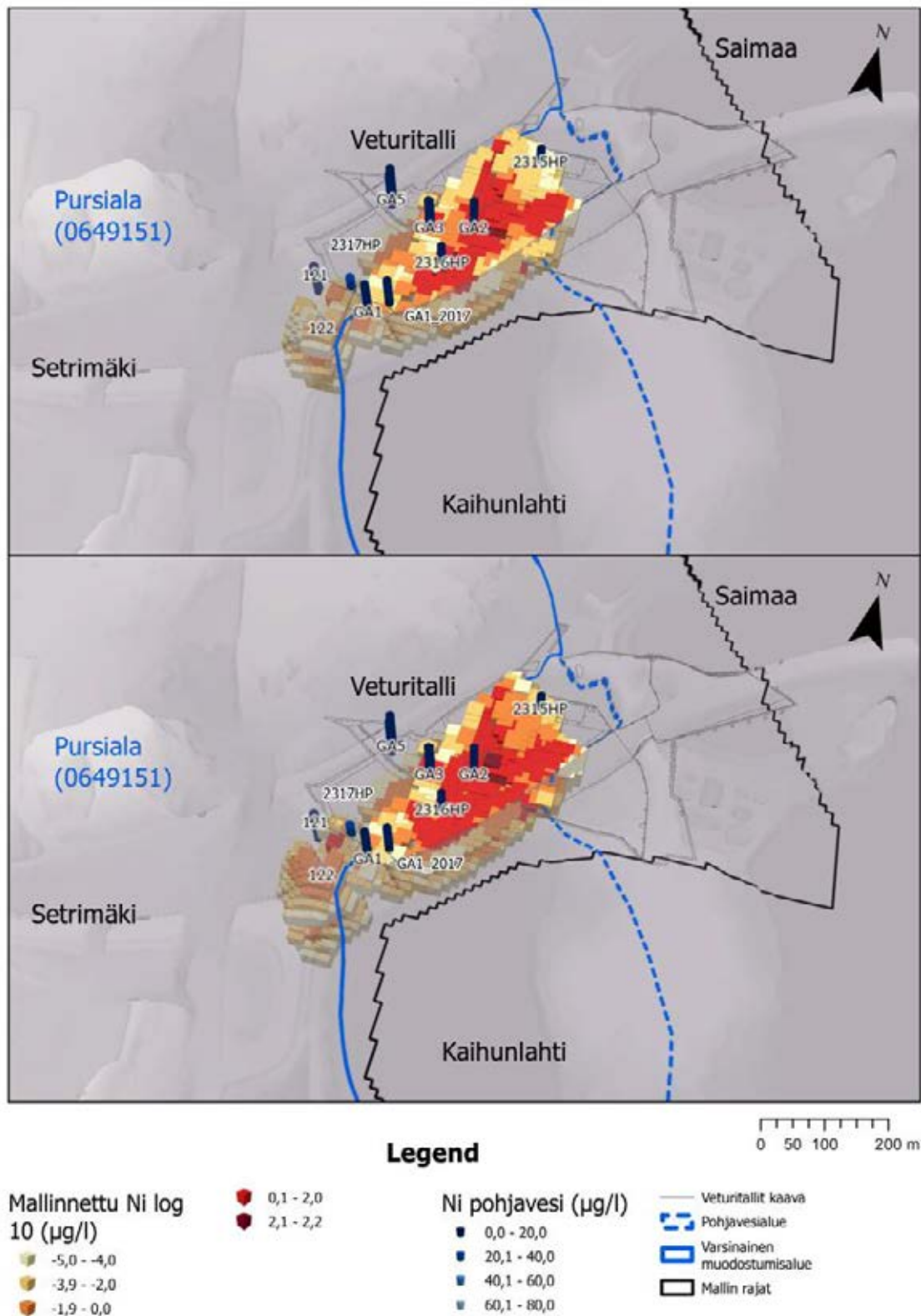
Kuva 4-10. Nikkelin pitoisuudet kuljetusmallin lähtötilassa (yllä). Nikkelin mallinnettu kulkeutuminen 60 vuoden kuluttua lähtötilanteesta (alla). Kuvan yksiköt ovat µg/l. Mallinnetut pitoisuudet ovat esitetty log 10 -muodossa niin, että esim. 2,0 vastaa arvoa 100 µg/l ja maksimiarvo on 170 µg/l. Vastaavasti -5 tarkoittaa pitoisuutta 0,00001 µg/l.
