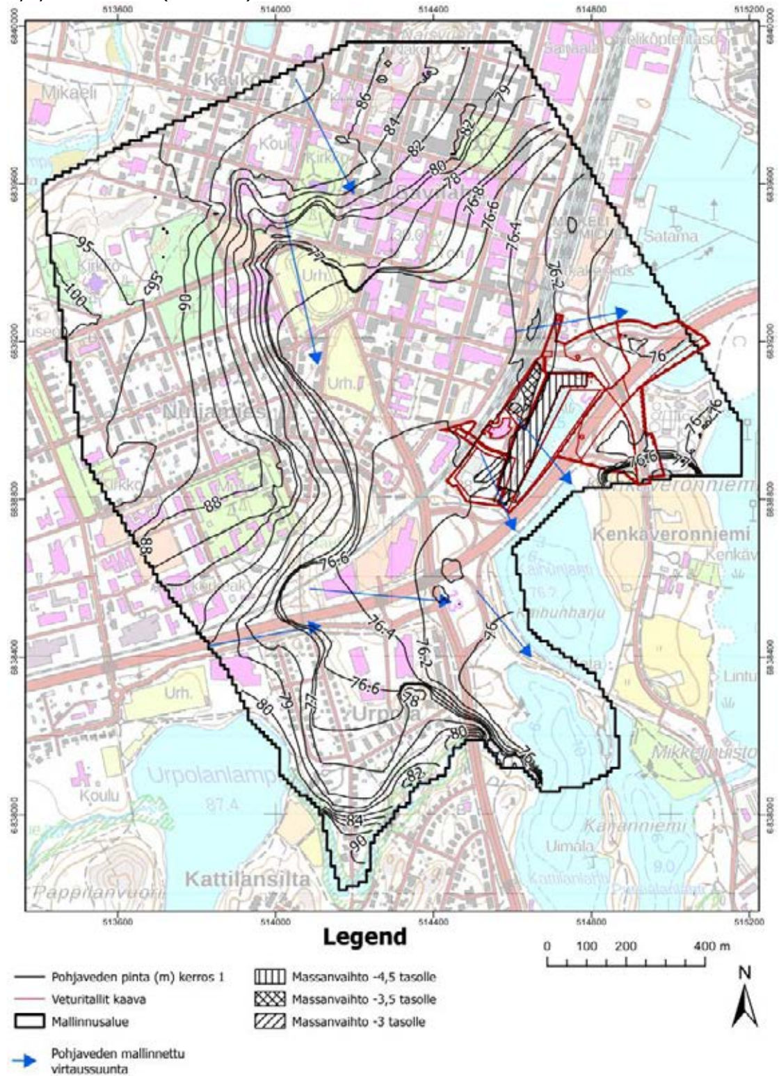
Kuva 4-4. Pohjaveden virtaussuunnat massanvaihdon tilanteen mallissa kerros 1:stä kuvattuna pohjaveden korkeuskäyrinä ja virtausnuolina (siniset nuolet).
