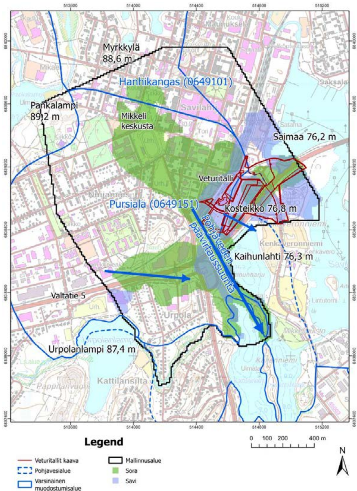
Kuva 1-1. Mallinnusalue, veturitallialueen suunnittelualue, pohjavesialueet ja lähialueiden pintavesien korkeustasot. Pohjaveden virtaussuunnat ovat esitetty sinisillä nuolilla. Kuvassa on myös esitettyä GTK:n 3d-malliin perustuvat rajaukset soralle ja savelle.
