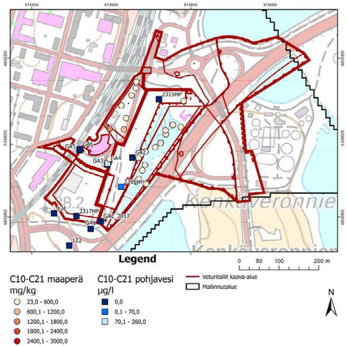
Kuva 3-8. Öljyn C10-C21 esiintyminen maaperässä ja pohjavedessä. Pohjaveden pitoisuudet ovat yksikössä µg/l ja maaperän mg/kg.
